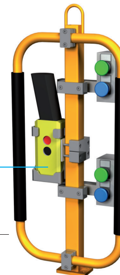
ERGO-Doppelhandlauf Hubtastensteuerung mit Greifer Tastensteuerung für: - Parallelspanner - Vakuumspanner - Magnetspanner
